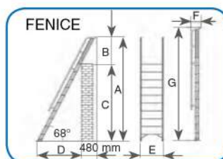
FENICE profondità gradino cm 10
