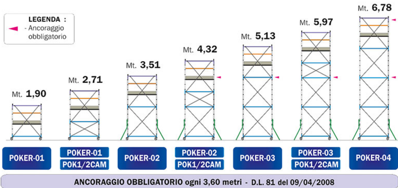
Configurazione POKER HD
