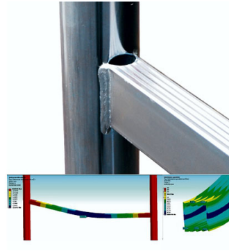
Gradino anti-scivolo ad alta resistenza
