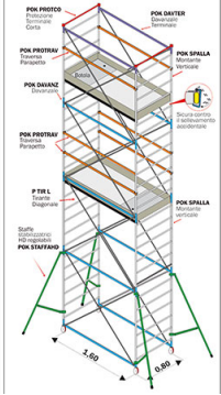
POKER HD disegno
