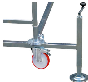
POR STAB V Stabilizzatori/livellatori a vite
