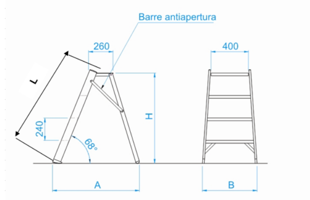
disegno tecnico
