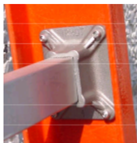
Particolare piolo
