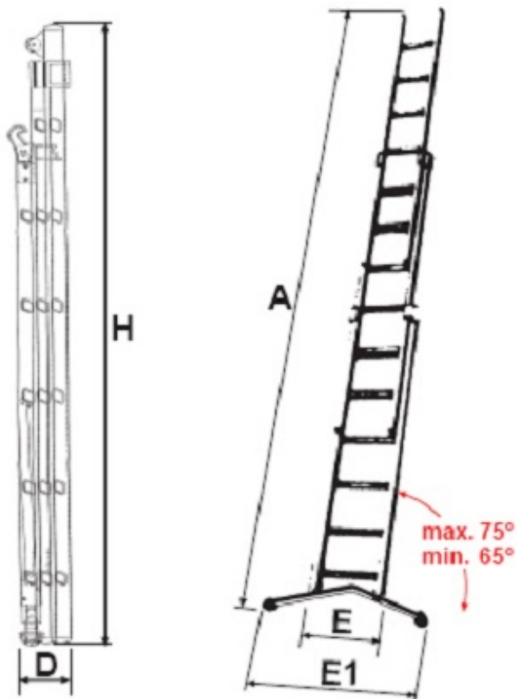
PRIMA a sfilo Disegno Tecnico
